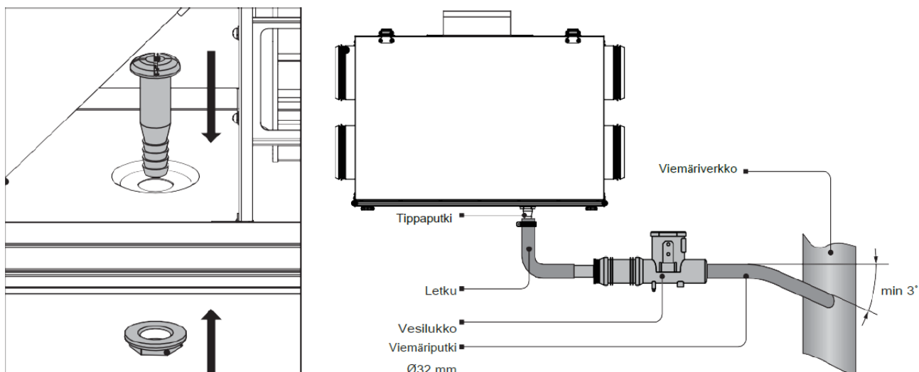
Kuva 3: Periaatekuva kondenssiveden viemäroinnistä
