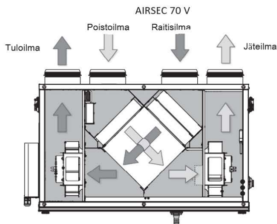
Kuva 2: Airsec 70 V ja 70 H toimintaperiaate
