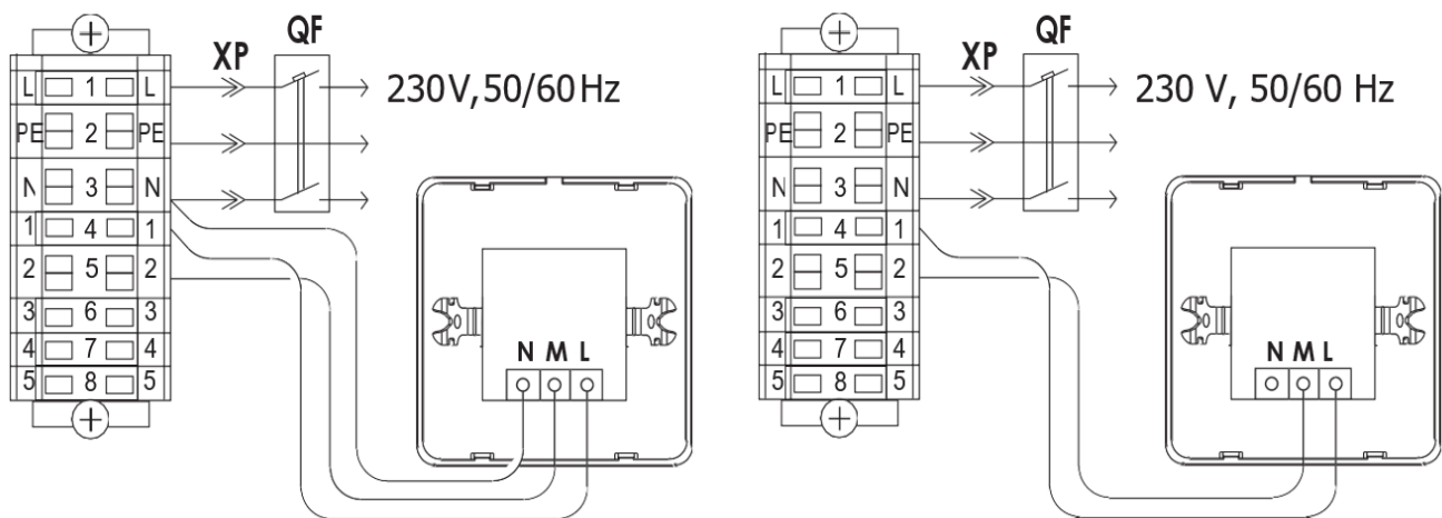
Kuva 4: Laitteen kytkentäkaavio
