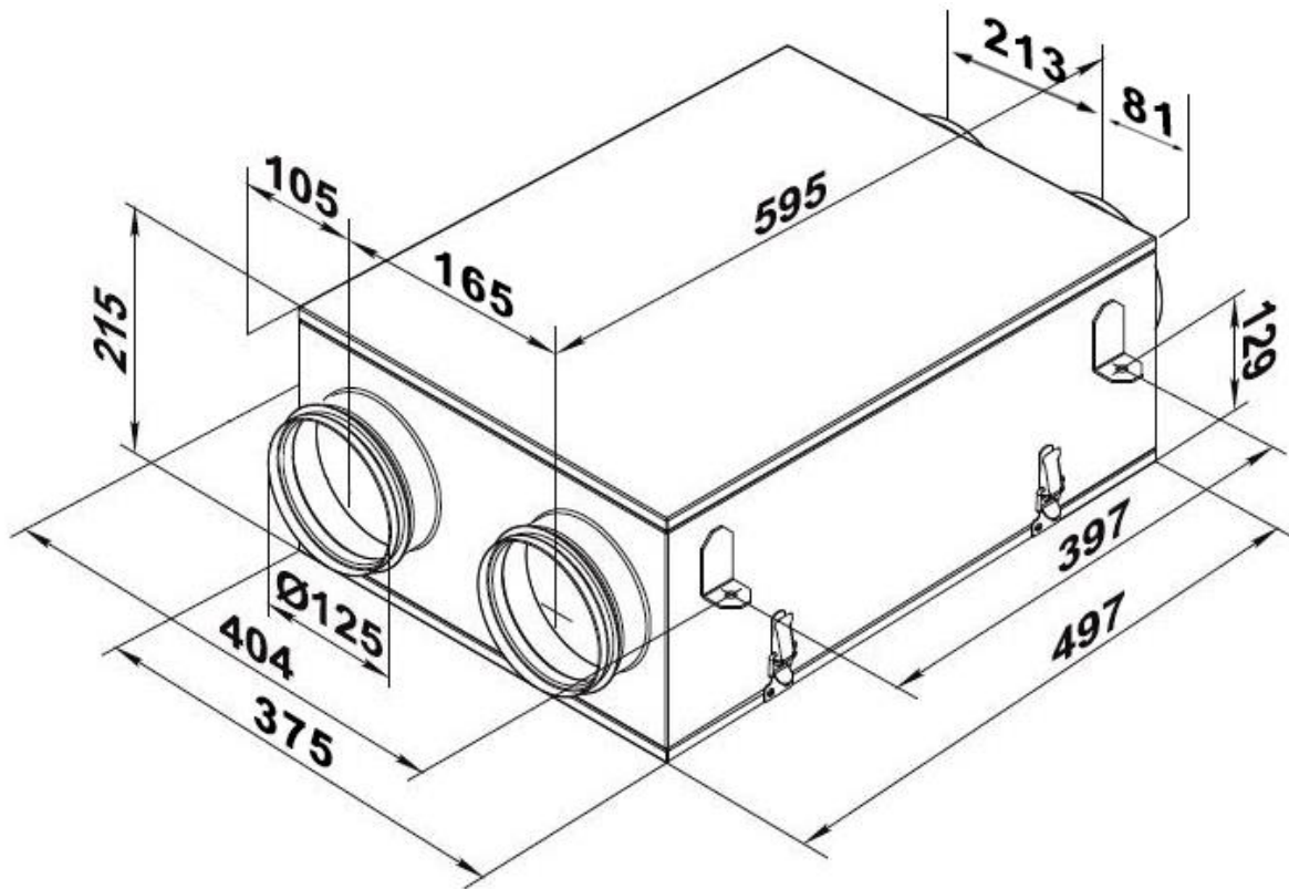
Kuva 1: Laitteen mitat (mm)
