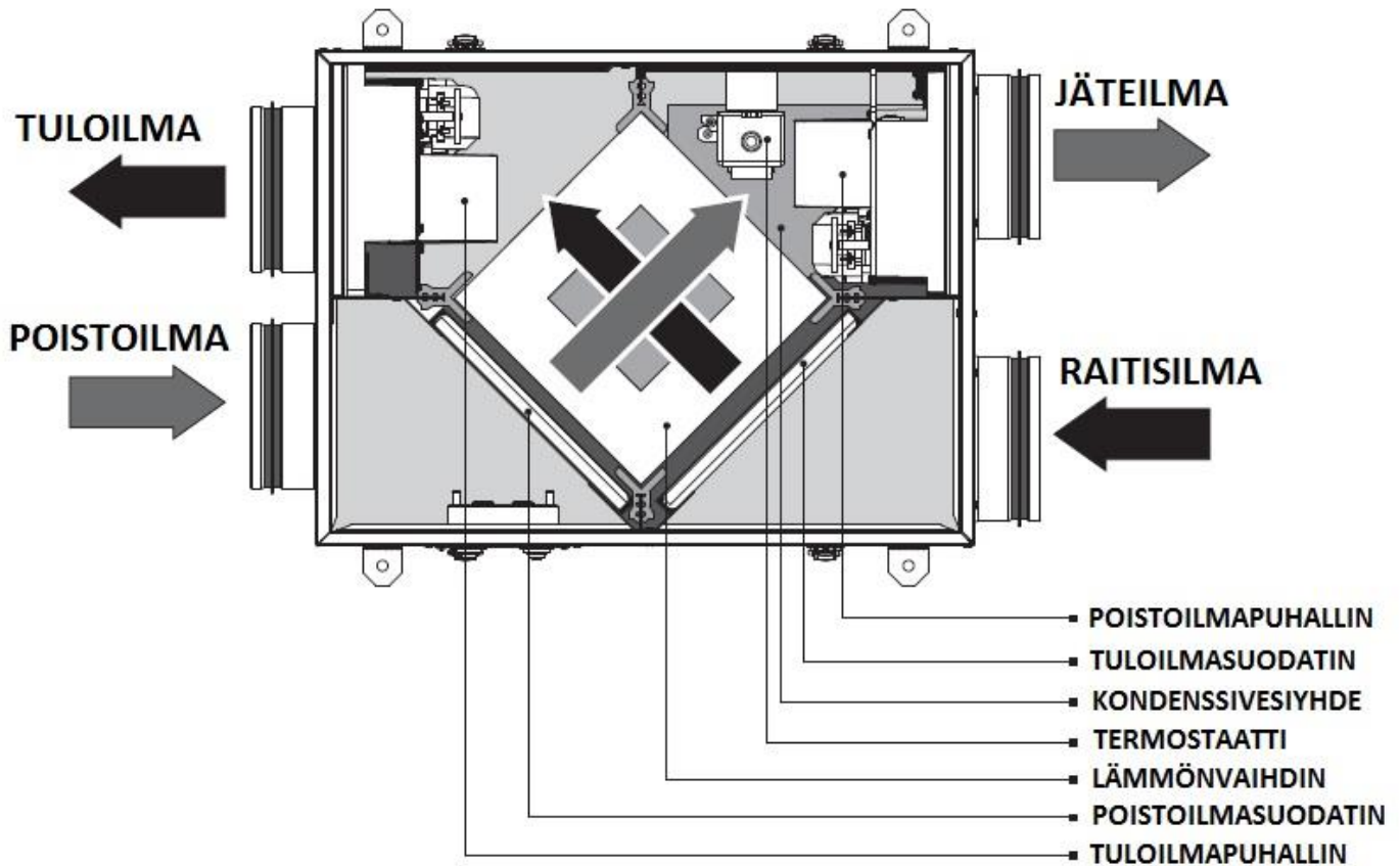
Kuva 2: Laitteen rakenne
