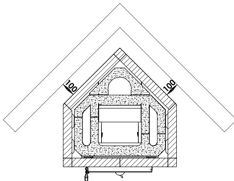
SECTION A-A SCALE 1 : 16
