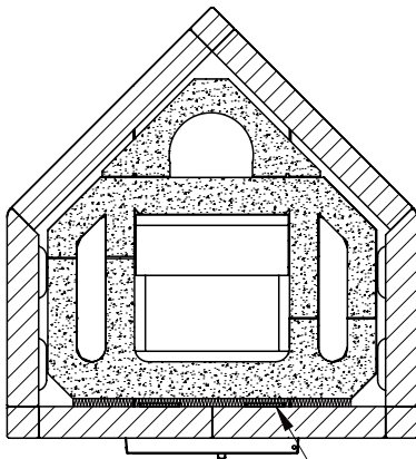
SECTION H-H SCALE 1 : 16 LUUKUN YLÄPUOLEN VILLA
