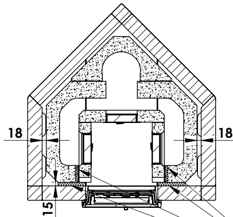
SECTION B-B SCALE 1 : 16
