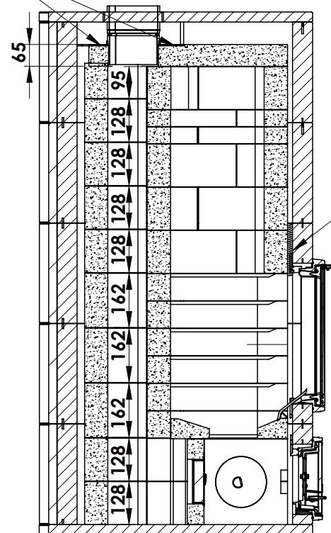
SECTION D-D SCALE 1 : 16
