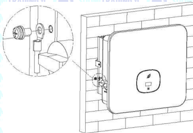
Figur 6.1 Jordningsdiagram
