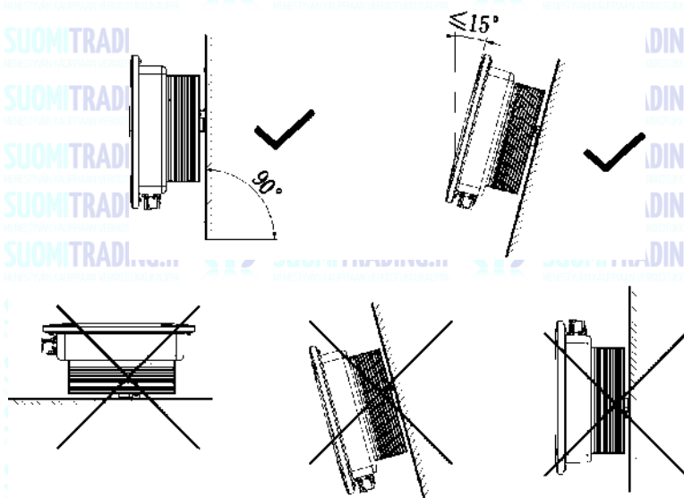
Figur 5.1 Installationsschema
