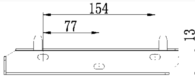
Kuva 5.7 Seinätelineen tiedot
