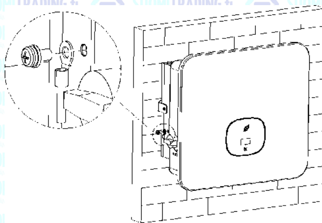
Figur 6.1 Jordningsdiagram
