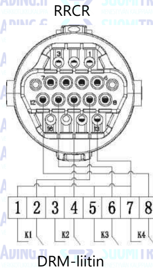
Kuva 6.20 Invertterin ja radiovärehtelyvastaanottimen (RRCR) kytkentä
