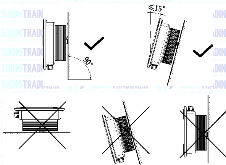
Figur 5.1 Installationsschema
