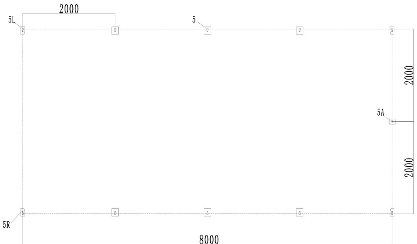
Kuva 2 Pohjalevy (yksikkö: mm)
